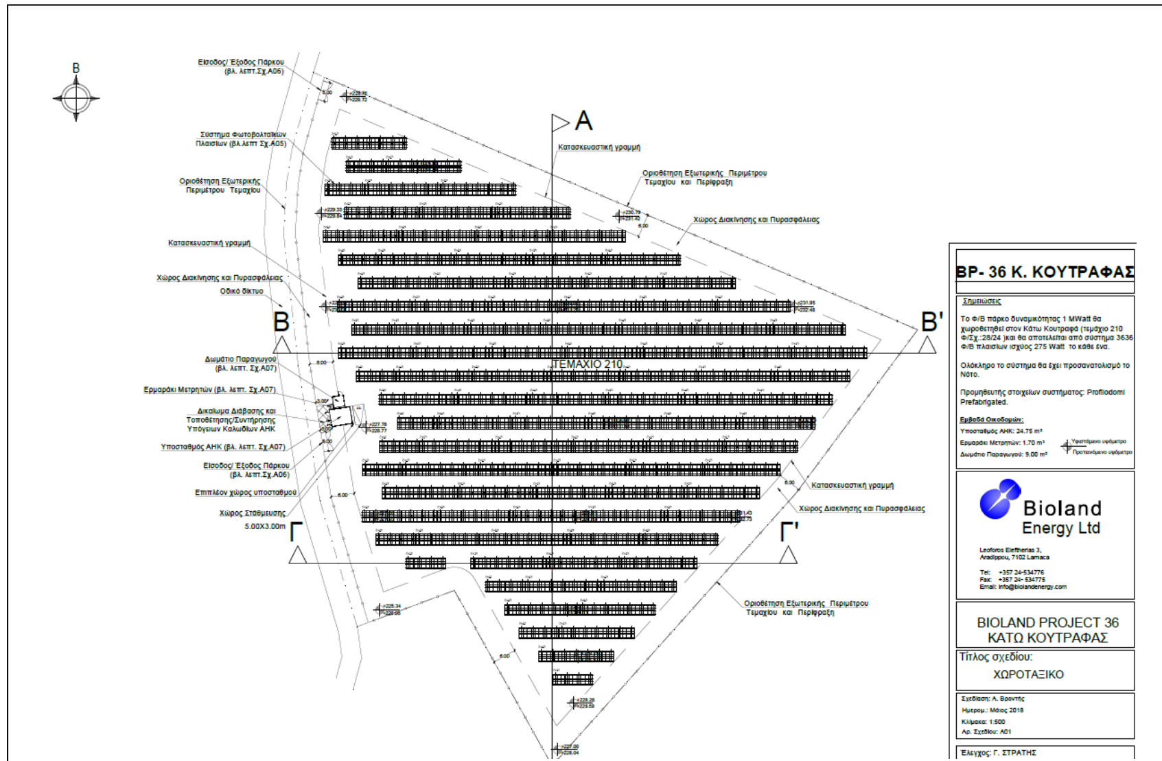
Εικόνα 2. Χωροταξικό σχέδιο του προτεινόμενου έργου.
