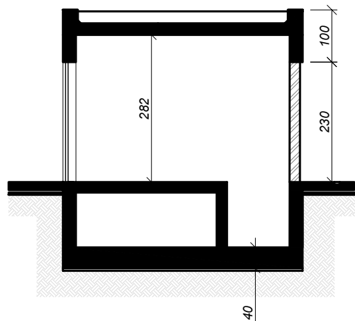
Τομή Δ'-Δ' ηλεκτρολογικών υποστατικών
