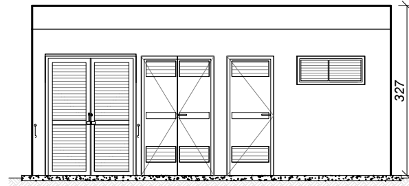
Όψη Α-Α' ηλεκτρολογικών υποστατικών
