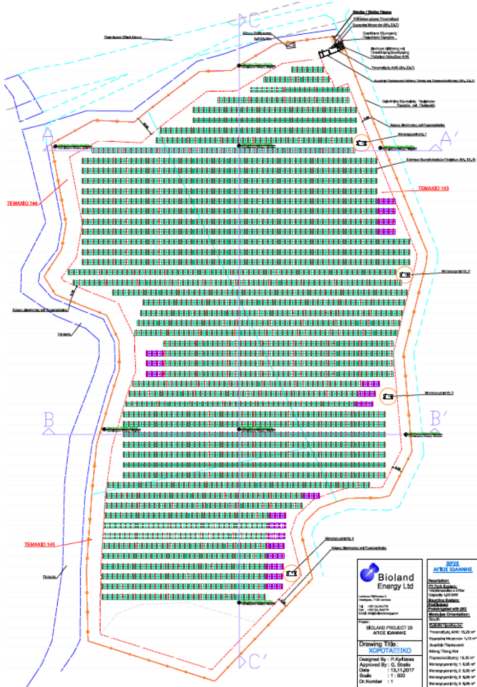
Εικόνα 2.3.1: Χωροταξικό σχέδιο προτεινόμενου έργου
