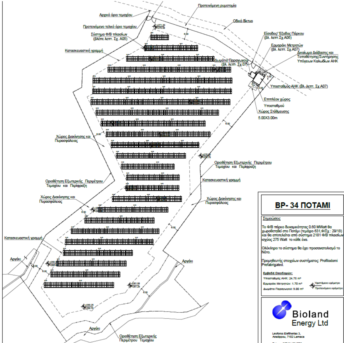
Εικόνα 2.3.1: Χωροταξικό σχέδιο προτεινόμενου έργου
