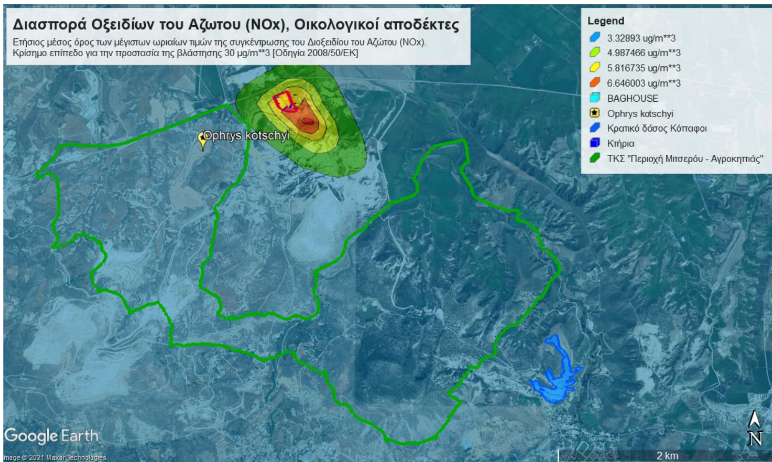
Εικόνα 4.15: Ετήσιος μέσος όρος των μέγιστων ωριαίων τιμών της συγκέντρωσης του Διοξειδίου του Αζώτου (NOx), οικολογικοί αποδέκτες
