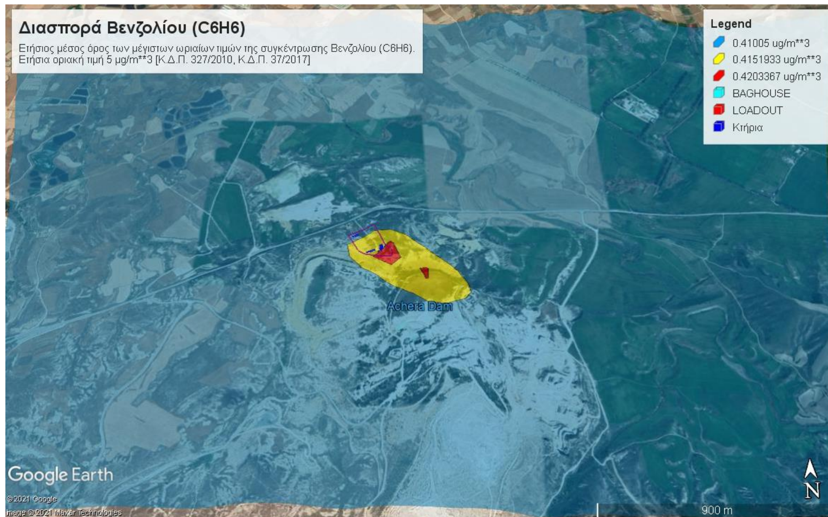
Εικόνα 4.12: Ετήσιος μέσος όρος των μέγιστων ωριαίων τιμών της συγκέντρωσης του Βενζολίου (C 6 H 6 )
