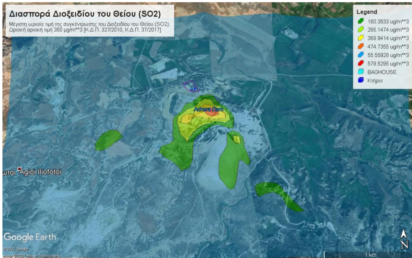
Εικόνα 4.4: Μέγιστη ωριαία τιμή της συγκέντρωσης του Διοξειδίου του Θείου (SO 2 )
