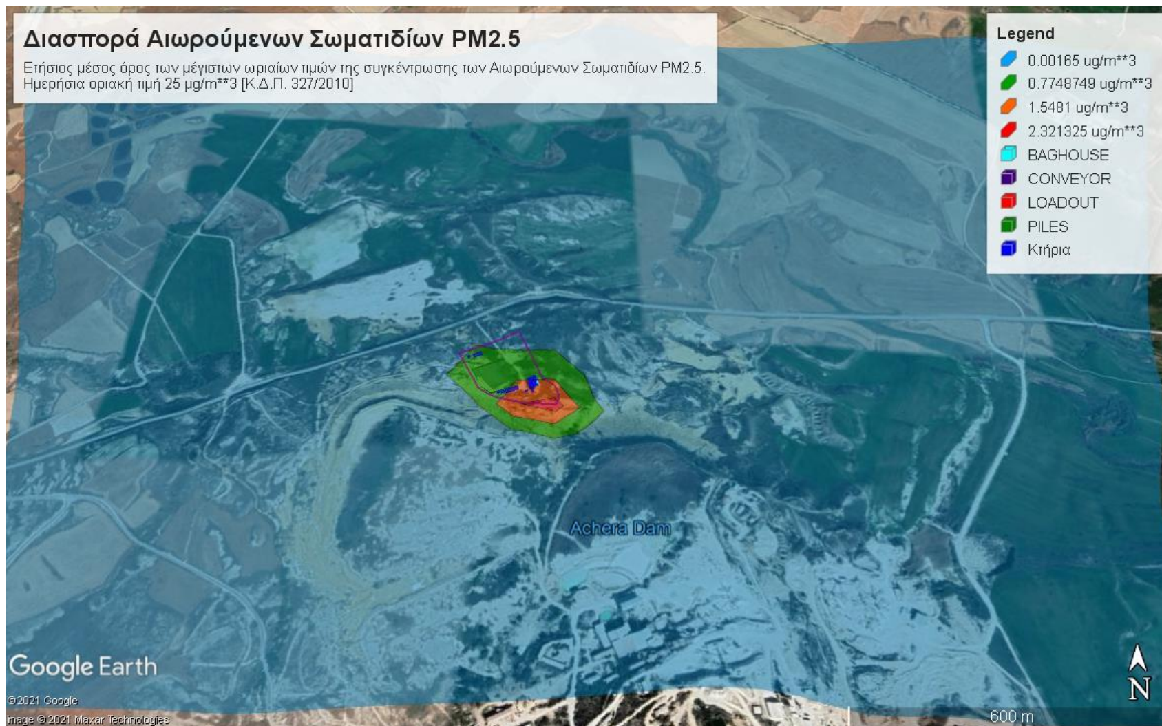
Εικόνα 4.3: Ετήσιος μέσος όρος των μέγιστων ωριαίων τιμών της συγκέντρωσης Αιωρούμενων Σωματιδίων 2.5 (PM 2.5 )
