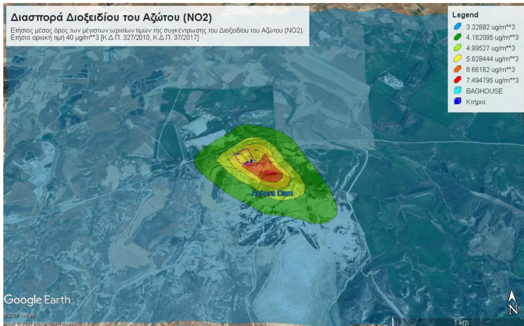
Εικόνα 4.7: Ετήσιος μέσος όρος των μέγιστων ωριαίων τιμών της συγκέντρωσης του Διοξειδίου του Αζώτου (NO 2 )
