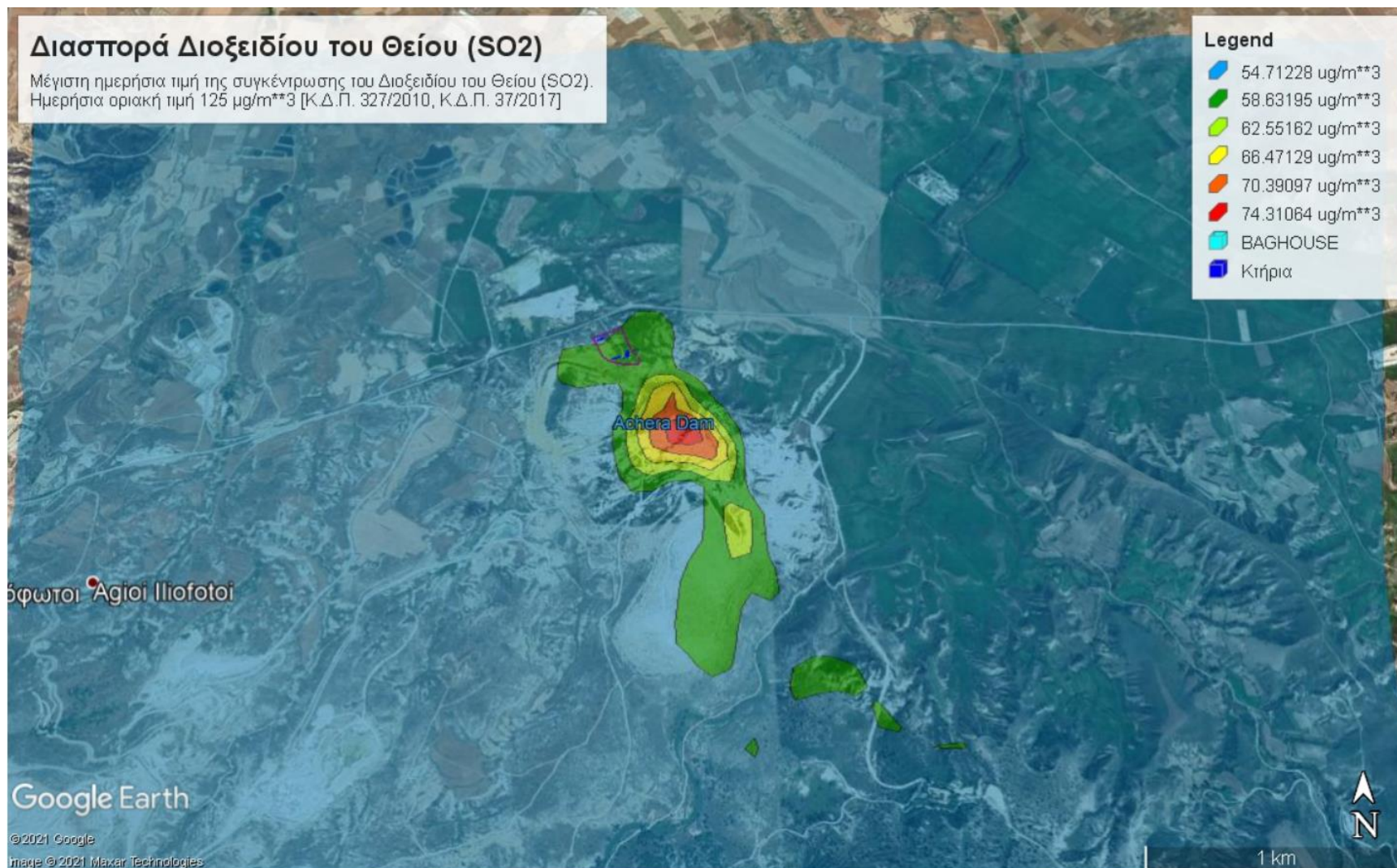
Εικόνα 4.5: Μέγιστη ημερήσια τιμή της συγκέντρωσης του Διοξειδίου του Θείου (SO 2 )
