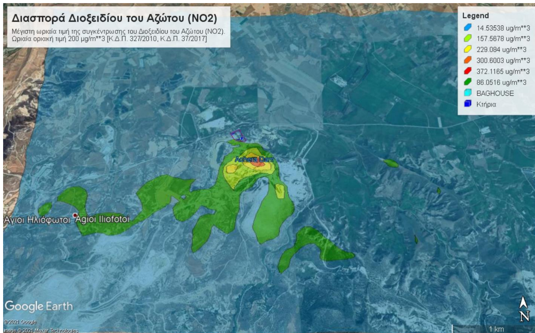
Εικόνα 4.6: Μέγιστη ωριαία τιμή της συγκέντρωσης του Διοξειδίου του Αζώτου (NO 2 )
