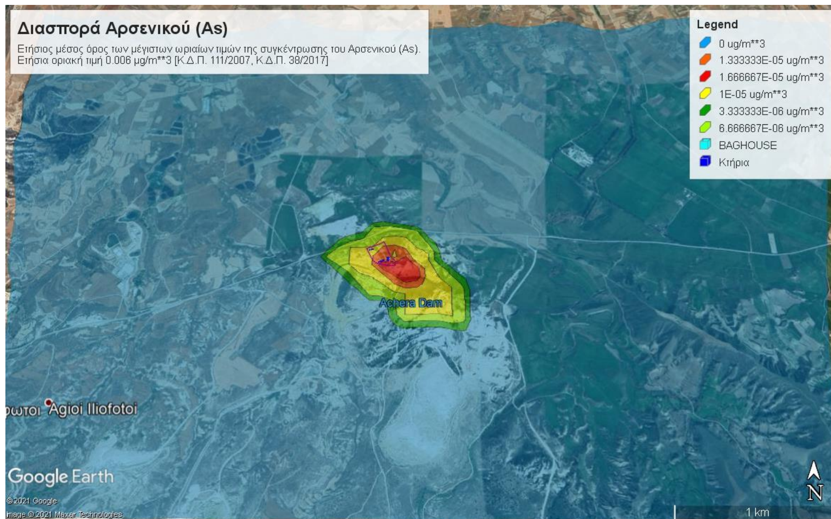
Εικόνα 4.9: Ετήσιος μέσος όρος των μέγιστων ωριαίων τιμών της συγκέντρωσης του Αρσενικού (As)
