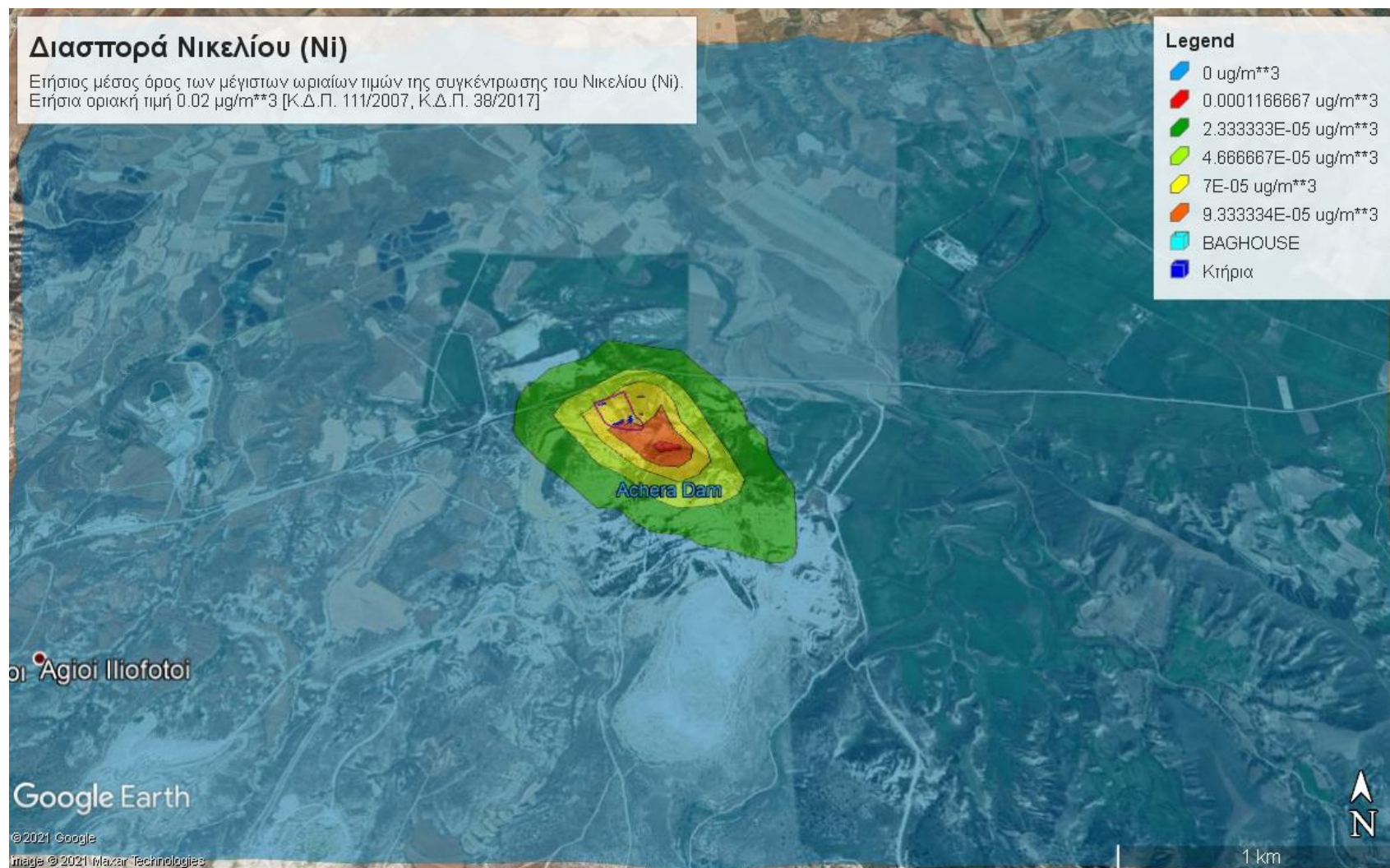
Εικόνα 4.11: Ετήσιος μέσος όρος των μέγιστων ωριαίων τιμών της συγκέντρωσης του Νικελίου (Ni)
