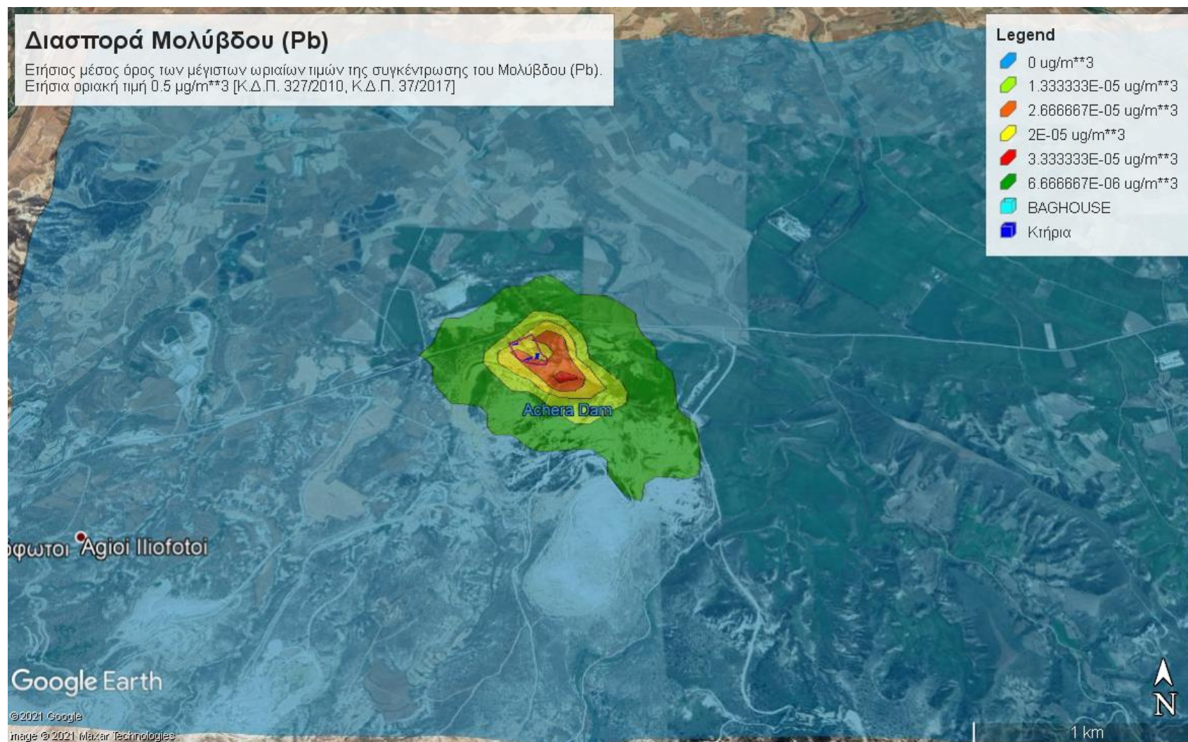
Εικόνα 4.8: Ετήσιος μέσος όρος των μέγιστων ωριαίων τιμών της συγκέντρωσης του Μόλυβδου (Pb)
