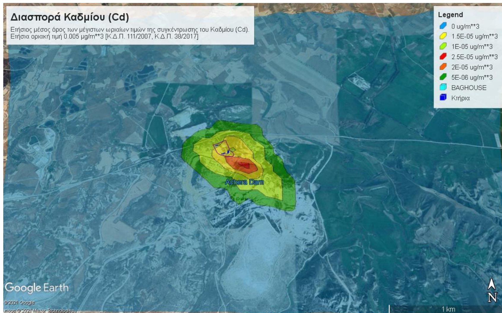
Εικόνα 4.10: Ετήσιος μέσος όρος των μέγιστων ωριαίων τιμών της συγκέντρωσης του Καδμίου (Cd)
