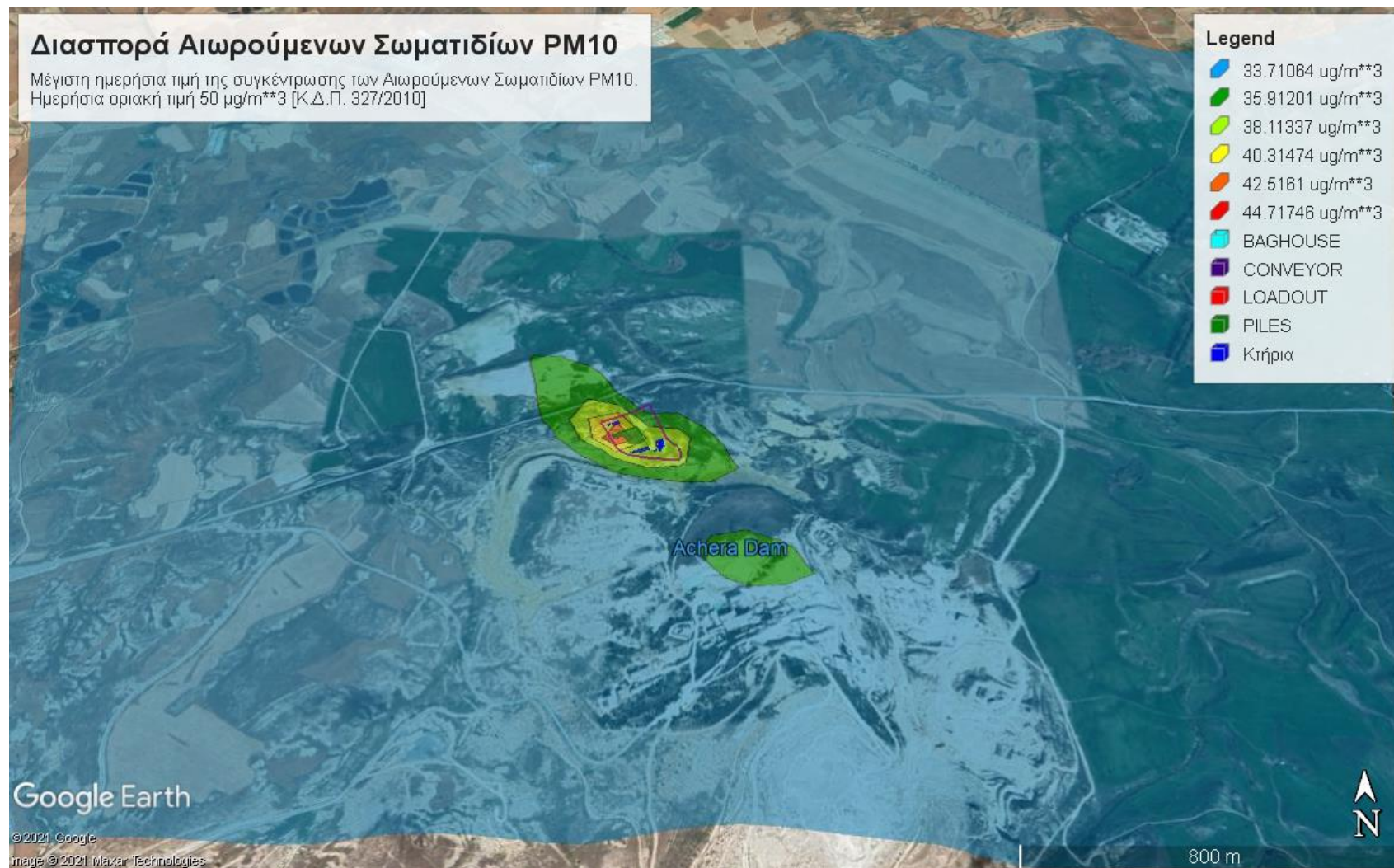
Εικόνα 4.1: Μέγιστη ημερήσια τιμή της συγκέντρωσης Αιωρούμενων Σωματιδίων 10 ( \text{PM}_{10} )
