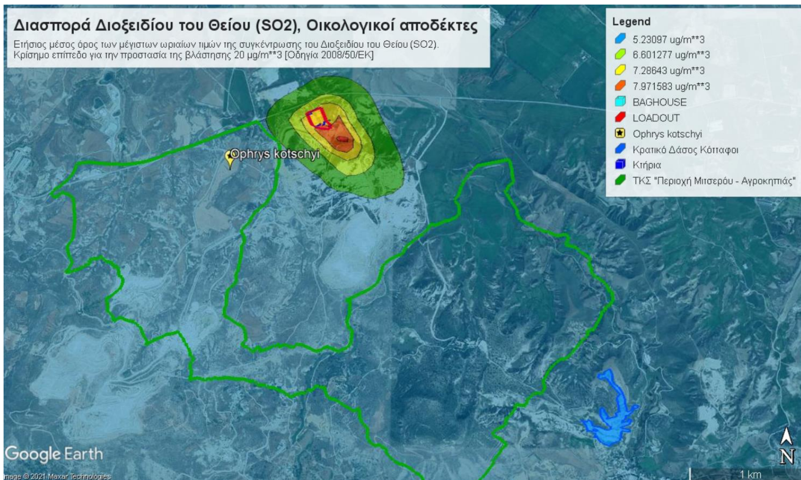
Εικόνα 4.14: Ετήσιος μέσος όρος των μέγιστων ωριαίων τιμών της συγκέντρωσης του Διοξειδίου του Θείου (SO 2 ), οικολογικοί αποδέκτες
