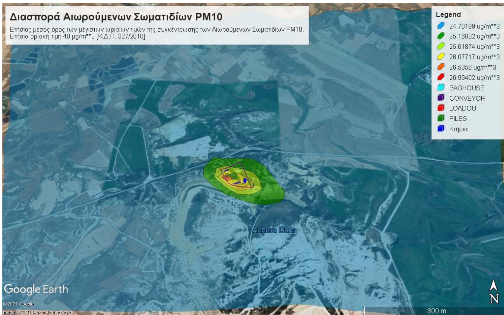
Εικόνα 4.2: Ετήσιος μέσος όρος των μέγιστων ωριαίων τιμών της συγκέντρωσης Αιωρούμενων Σωματιδίων 10 (PM 10 )
