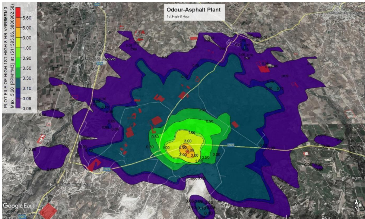
Σχήμα 10: Συγκεντρώσεις οσμών από το ασφαλτικό-1 η μέγιστη οκτάωρη συγκέντρωση.
