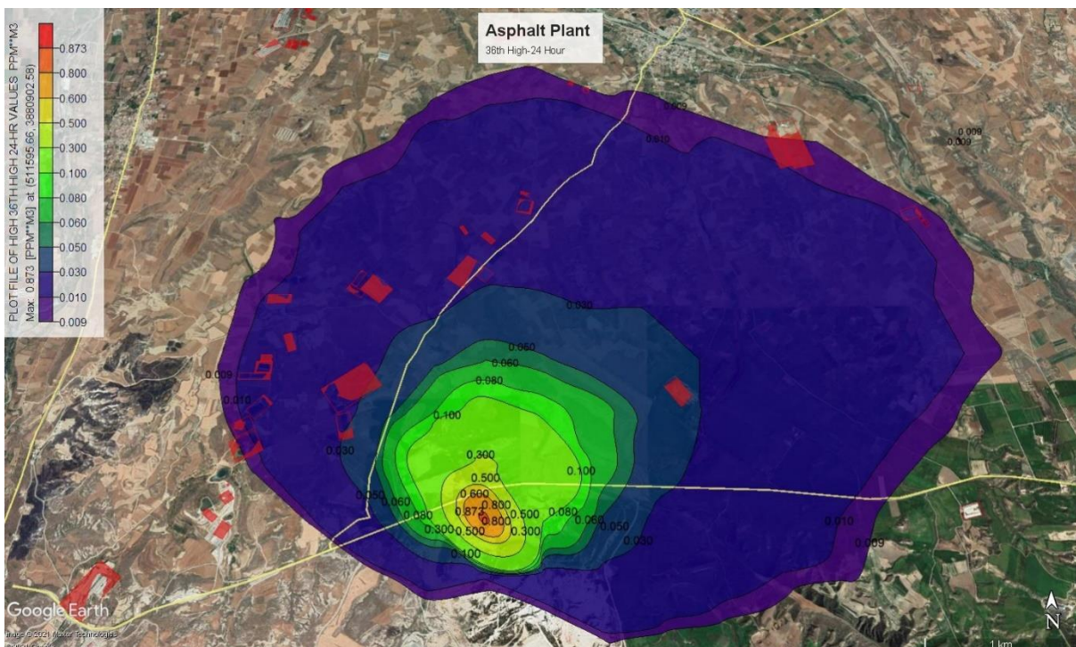
Σχήμα 14: Συγκεντρώσεις οσμών από το ασφαλτικό - χειρότερη (98 ο εκατοστημόριο) μέγιστη ημερησια συγκέντρωση.
