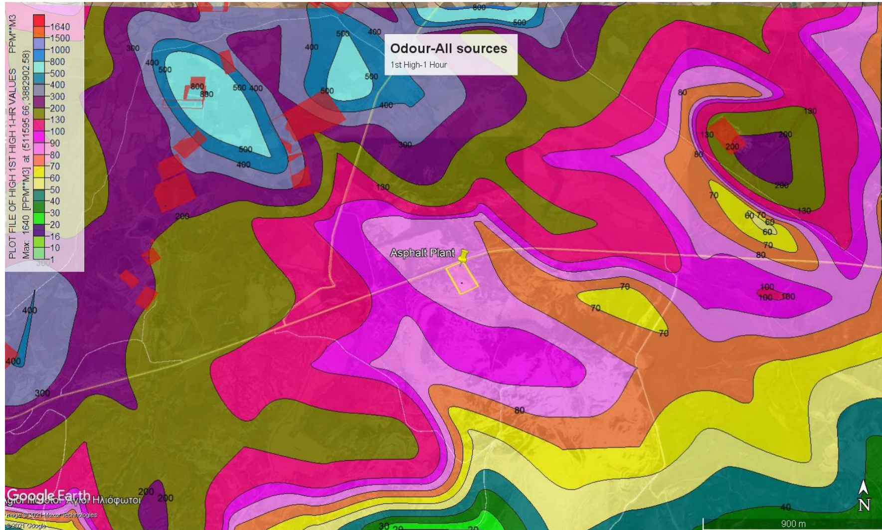
Σχήμα 16: Συγκεντρώσεις οσμών από το ασφαλτικό και τις οχηματικές εγκαταστάσεις-1 η ωριαία μέγιστη συγκέντρωση στην περιοχή του ασφαλτικού.
