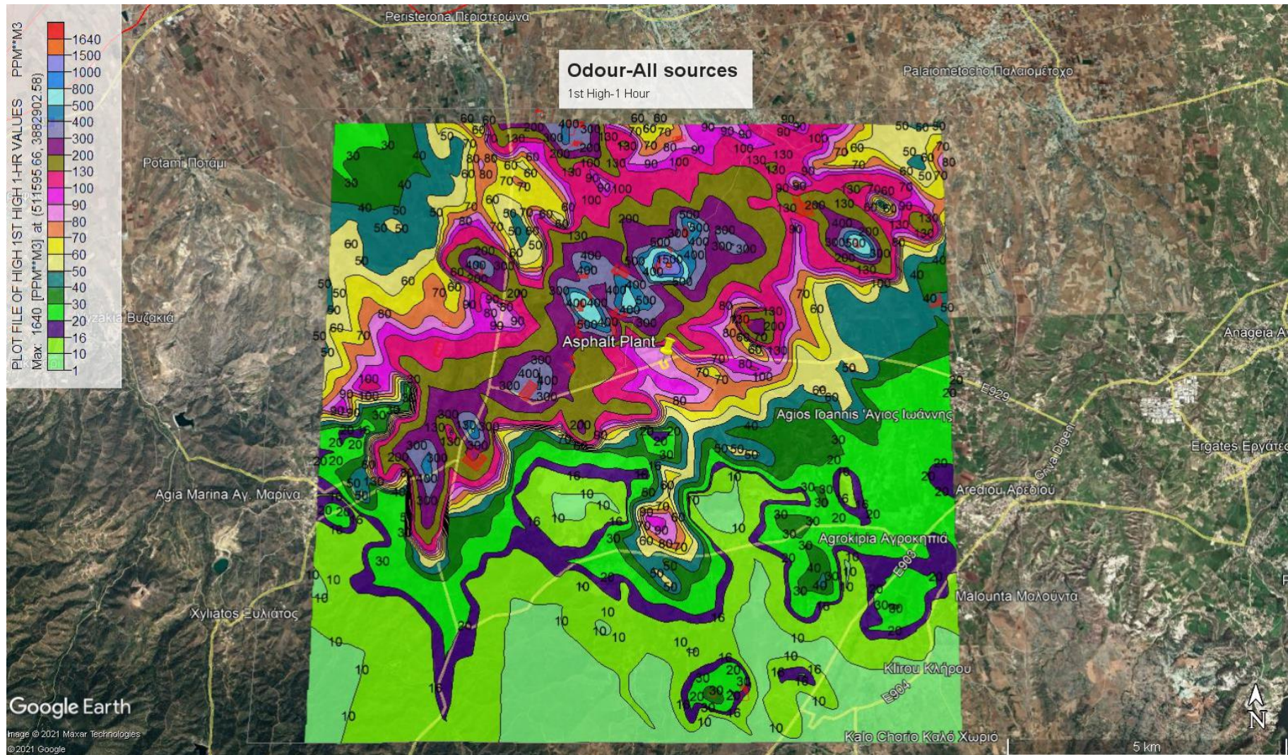
Σχήμα 15: Συγκεντρώσεις οσμών από το ασφαλτικό και τις οχληρές εγκαταστάσεις-1 η ωριαία μέγιστη συγκέντρωση.
