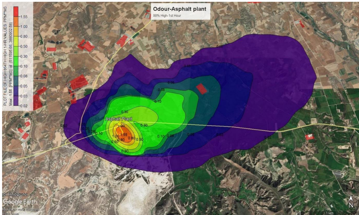
Σχήμα 12: Συγκεντρώσεις οσμών από το ασφαλτικό -χειρότερη (98 ο εκατοστημόριο) μέγιστη ωριαία συγκέντρωση.
