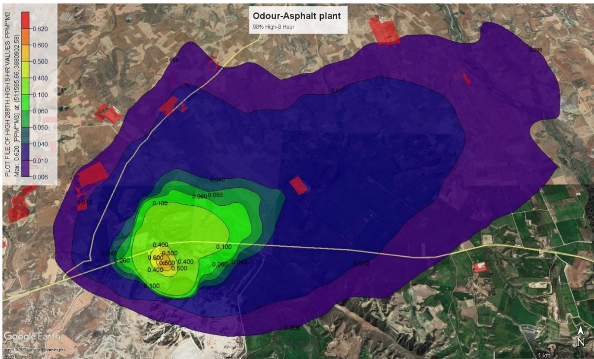
Σχήμα 13: Συγκεντρώσεις οσμών από το ασφαλτικό - χειρότερη (98 ο εκατοστημόριο) μέγιστη οκτάωρη συγκέντρωση.
