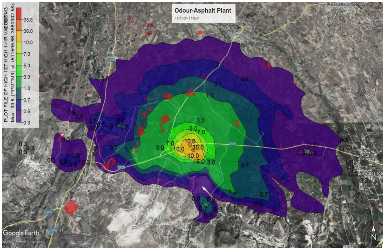
Σχήμα 9: Συγκεντρώσεις οσμών από το ασφαλτικό - 1 η μέγιστη ωριαία συγκέντρωση.
