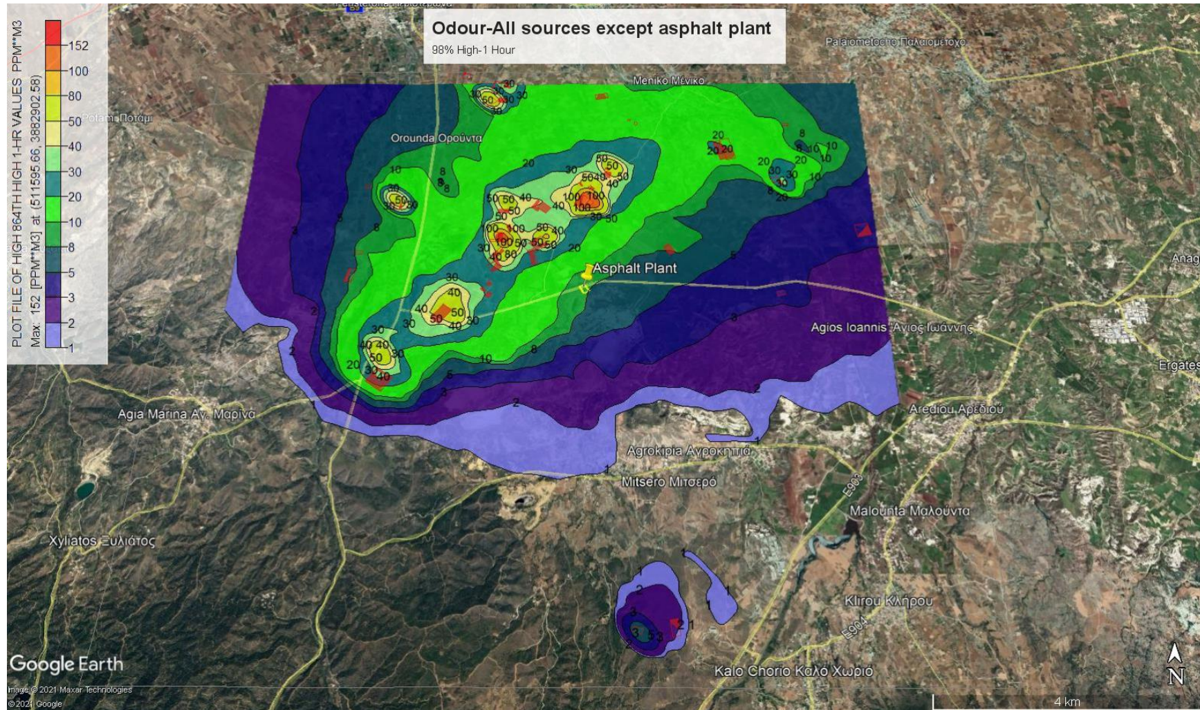
Σχήμα 7: Συγκεντρώσεις οσμών από οχληρές εγκαταστάσεις εκτός του ασφαλτικού- Χειρότερη (98 ο εκατοστημόριο) μέγιστη ωριαία συγκέντρωση .
