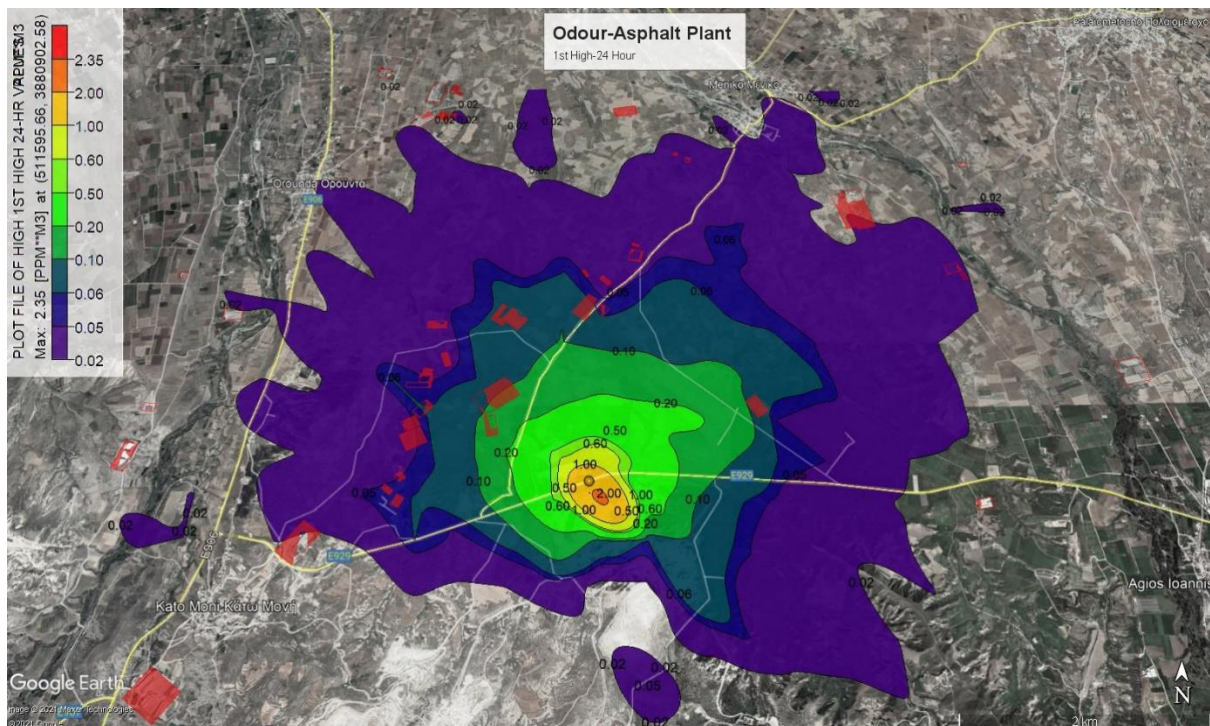
Σχήμα 11: Συγκεντρώσεις οσμών από το ασφαλτικό-1 η μέγιστη ημερήσια συγκέντρωση.
