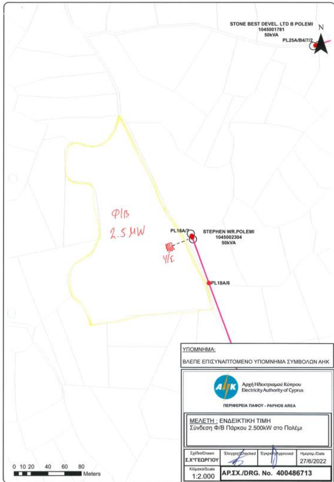
Εικόνα 6: Ο προτεινόμενος τρόπος σύνδεσης του Αγρο φωτοβολταϊκού πάρκου με το δίκτυο της ΑΗΚ.
