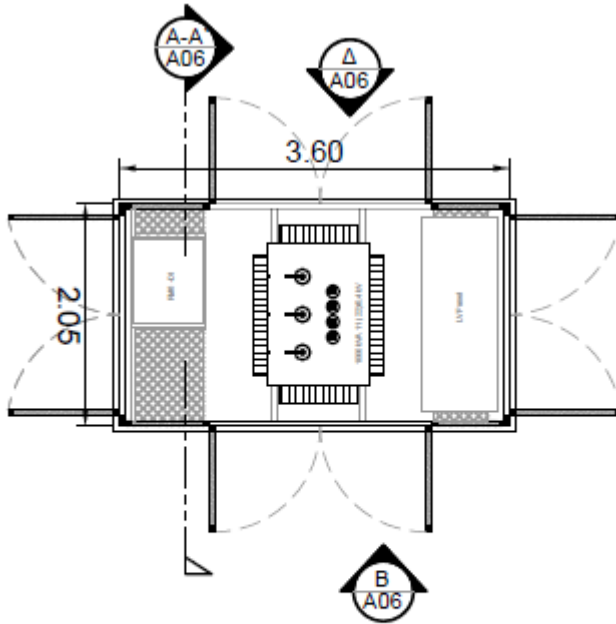
ΣΧ.5 ΚΑΤΟΨΗ ΔΩΜΑΤΙΟΥ Μ/Σ A06 1:100
